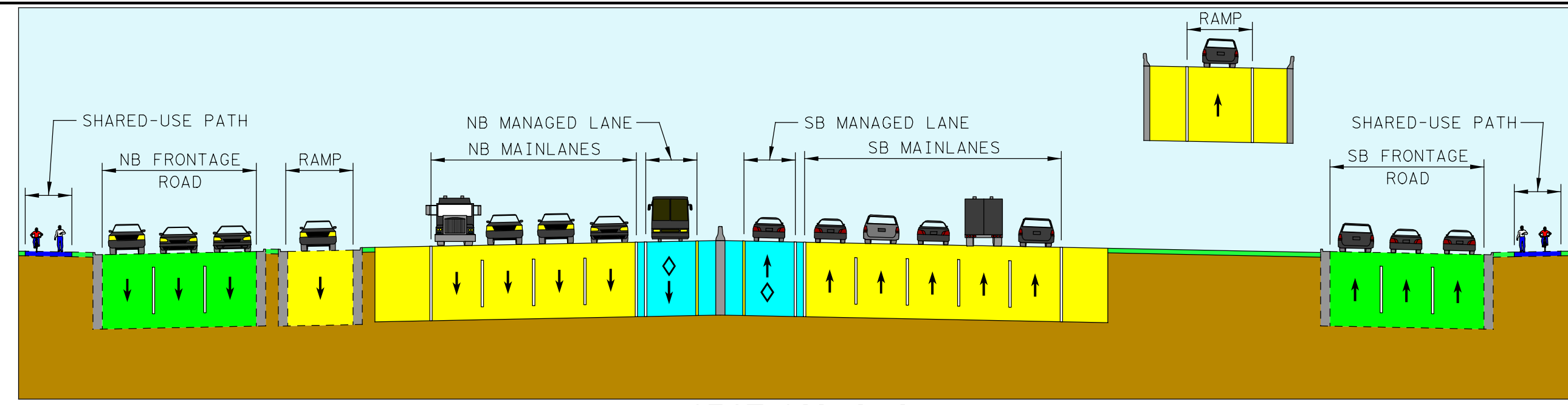
SECTION A-A
